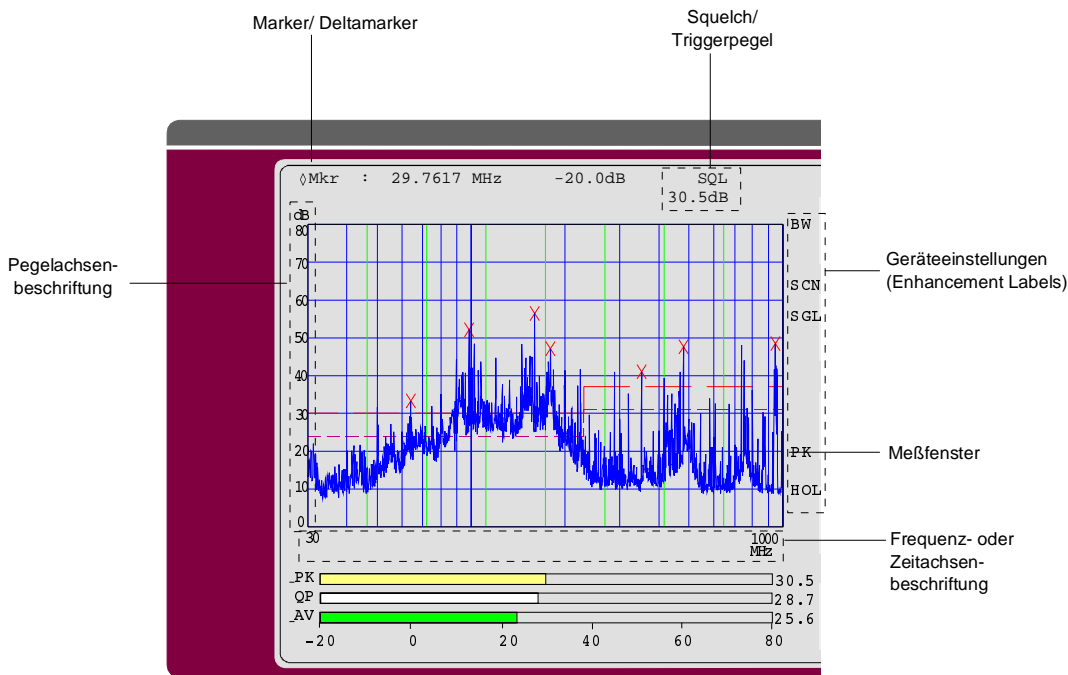
Bild 3-3 Bildschirmaufteilung des ESCS
