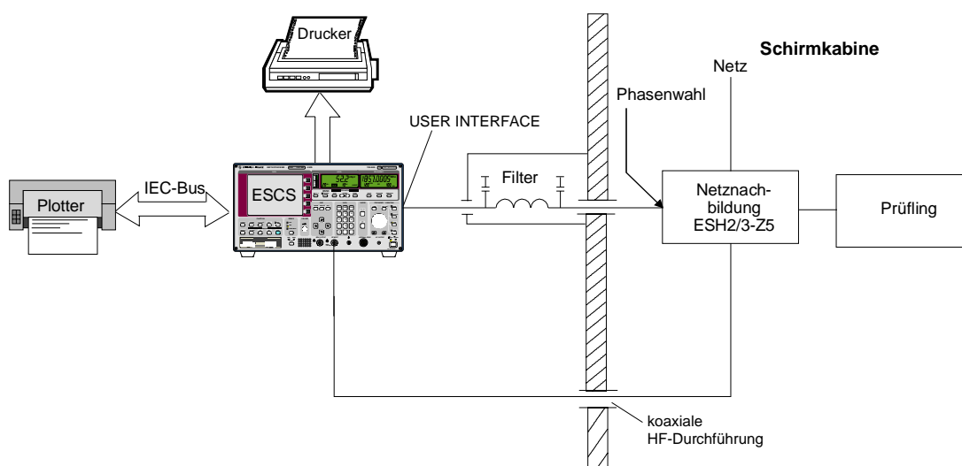
Bild 2-1 Blockschaubild eines Meßaufbaus mit Netznachbildung und Prüfling in einer geschirmten Kabine
