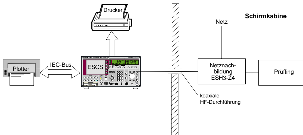
Bild 2-7 Blockschaubild eines Meßaufbaus mit Netznachbildung und Prüfling in einer geschirmten Kabine
