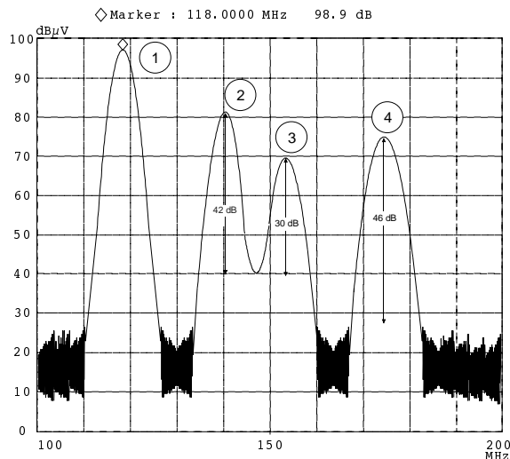
Bild 4-11 Beispiel für verschiedenen Einstellungen von Peak Excursion
