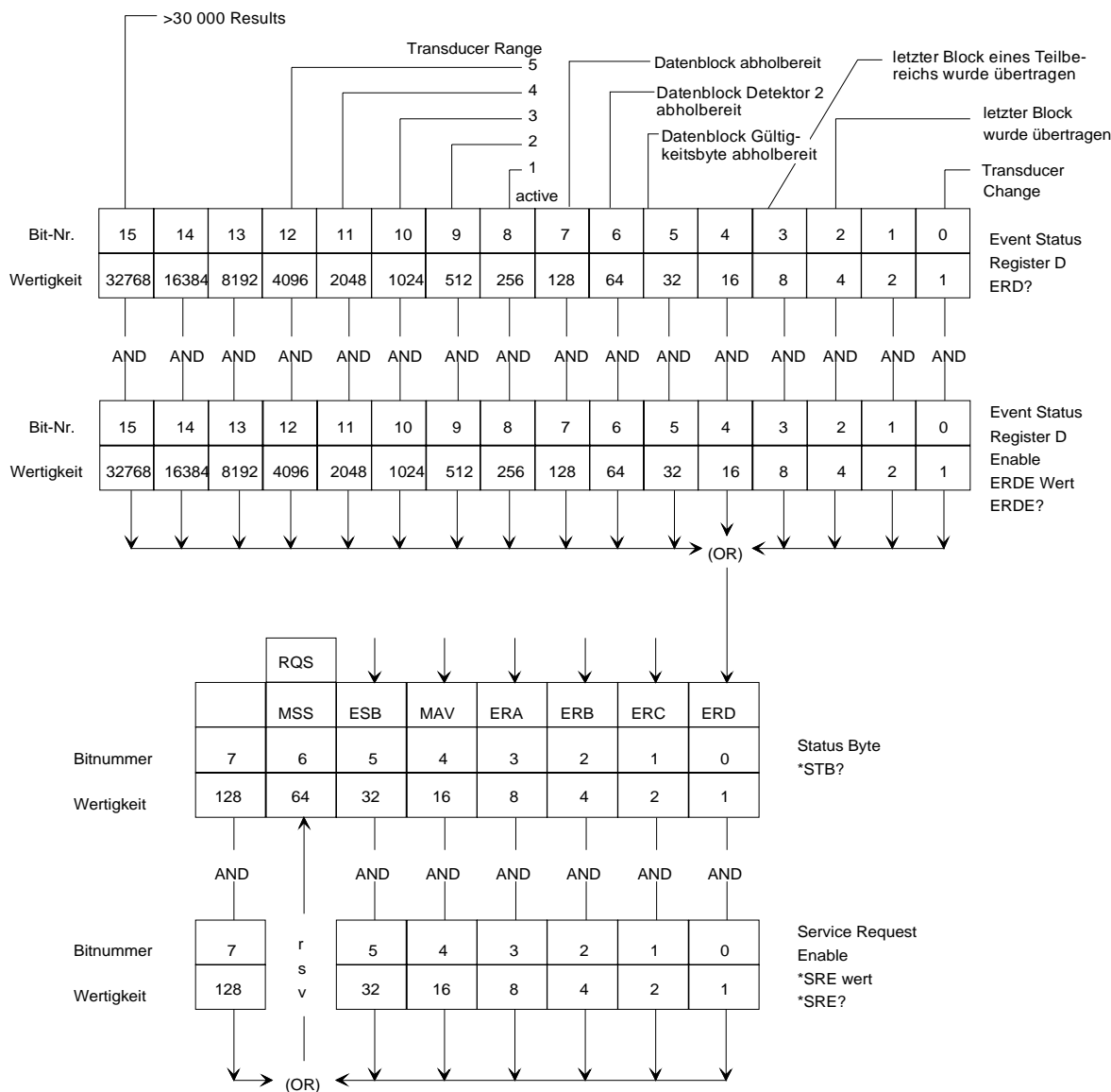
Bild 6-6 Statusregister ERD
